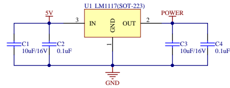
LDO
