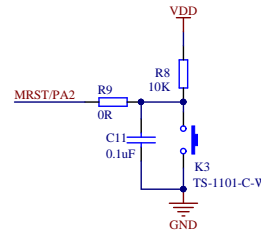
RSET
