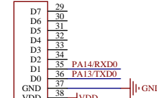
ARDUINO_INTERFACE
