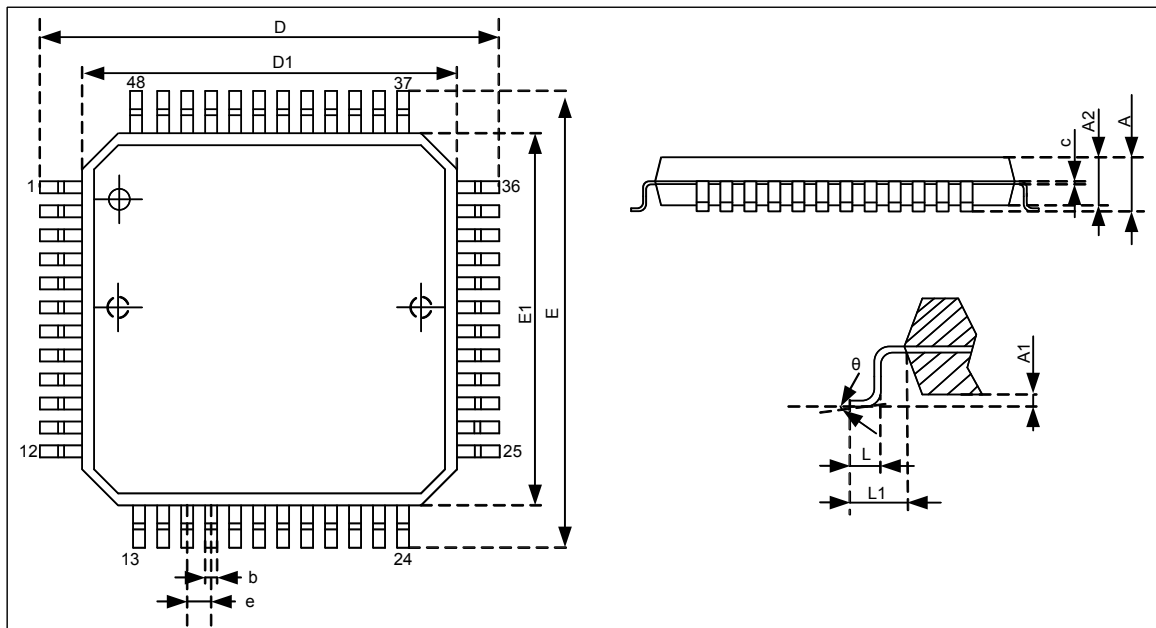
LQFP48
