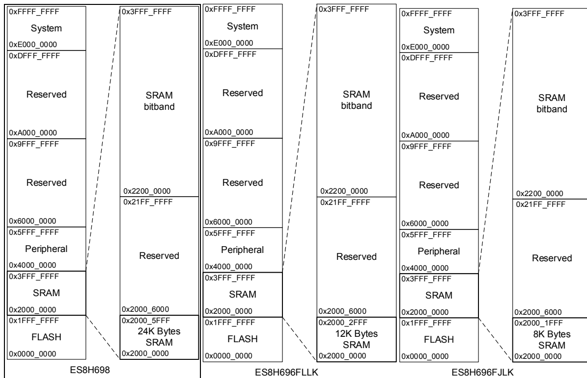
图 3-8 SRAM 映射图
