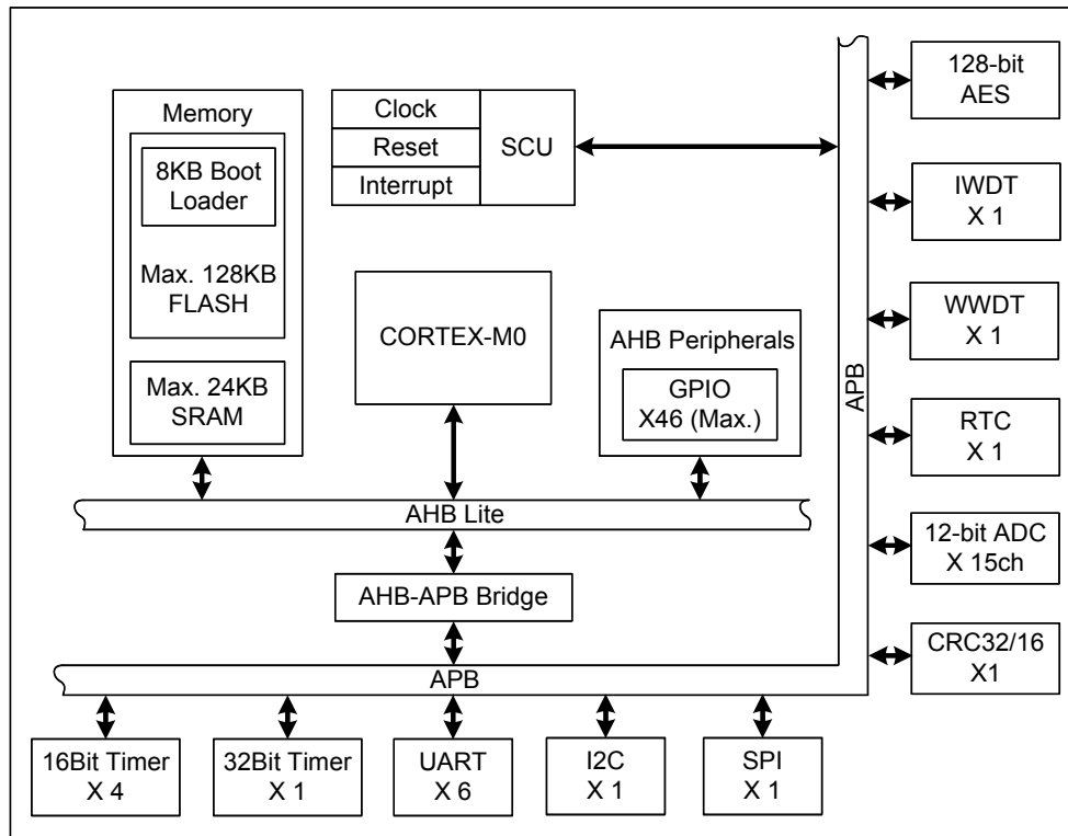
图 1-1 ES8H69x 结构框图
