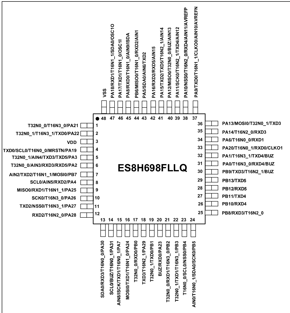
图 1-3 ES8H698FLLQ LQFP48 封装顶视图
