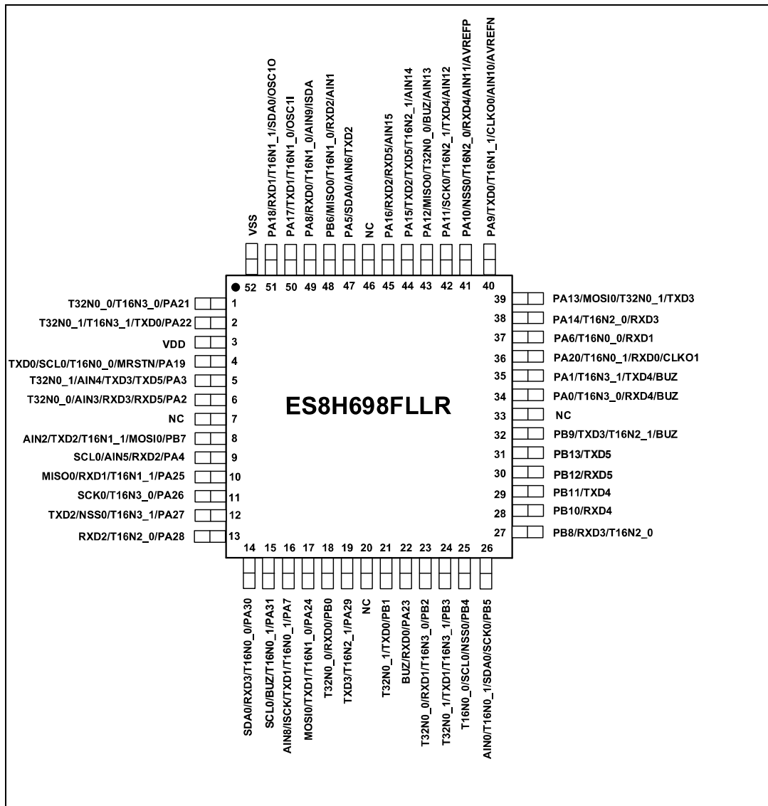
图 1-2 ES8H698FLLR LQFP52 封装顶视图
