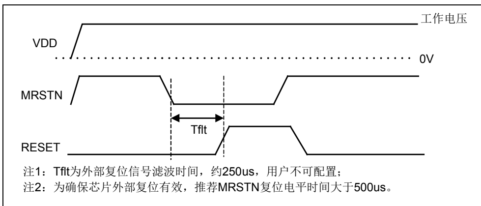
图 2-5 外部复位时序示意图
