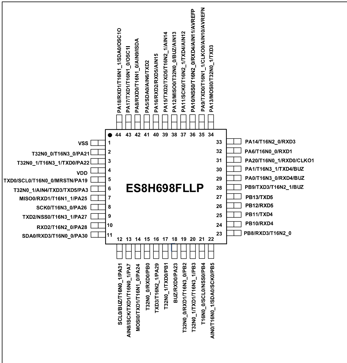
图 1-4 ES8H698FLLP LQFP44 封装顶视图
