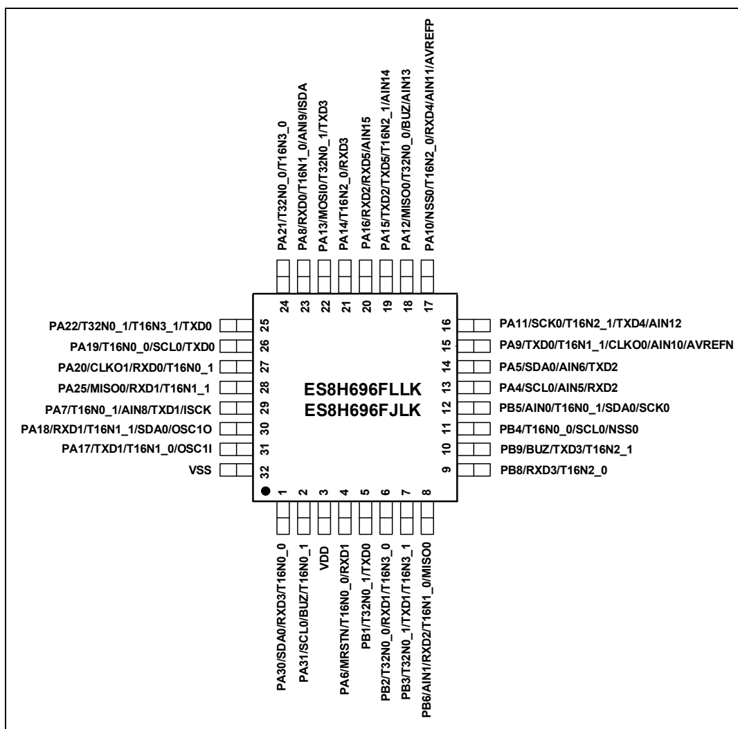
图 1-5 ES8H696FJLK/ES8H696FLLK LQFP32 封装顶视图
